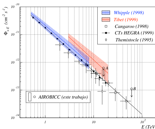
Fig. 1. Espectro de muy alta energía de la nebulosa del Cangrejo. Se muestran los resultados obtenidos con AIROBICC junto a los de otros autores.
