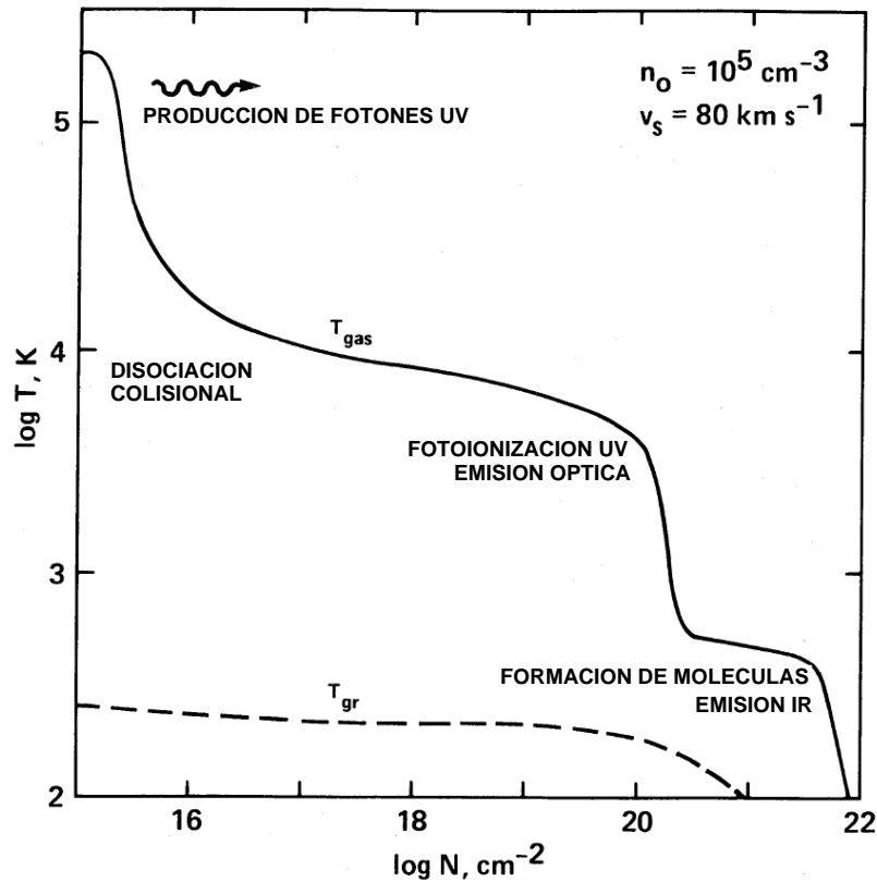
FIGURA 2.6: Diferentes regiones de los choques tipo-J. Figura de Hollenbach & McKee (1989).
