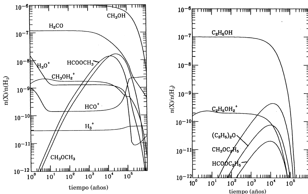
FIGURA 2.7: Modelos en los que se representa la química en fase gaseosa a partir del \text{CH}_3\text{OH} y del \text{C}_2\text{H}_5\text{OH} . Figura adaptada de Charnley et al. (1995).
