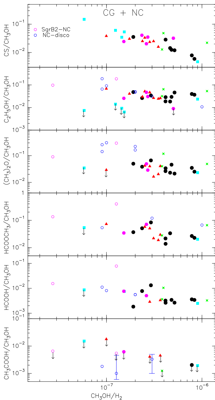
FIGURA 3.9: En esta figura se presentan las razones de abundancias para las nubes del CG y las que se encuentran en los núcleos calientes. Los datos de los núcleos calientes han sido obtenidos de Ikeda et al. (2001) y Remijan et al. (2002, 2003). Ver Fig. 3.6.
