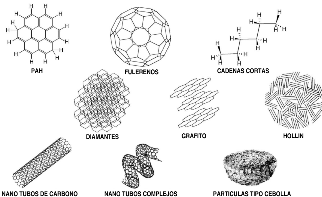
FIGURA 2.8: Moléculas gigantes formadas por carbonos. Figura adaptada de Ehrenfreund & Charnley (2000).
