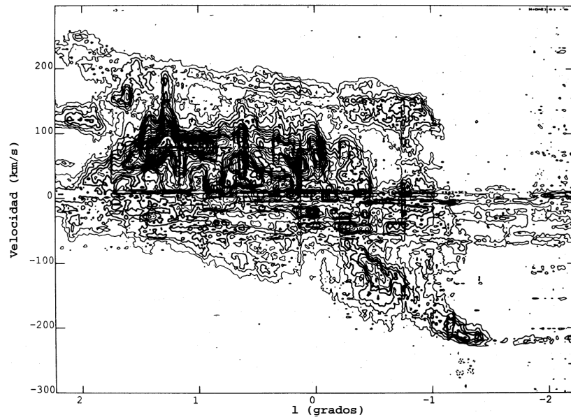
FIGURA 1.5: Diagrama de distribución de velocidades de la emisión de CO de Bally et al. (1987) para el intervalo de latitud |b| < 0^\circ.1 . Los contornos representan la intensidad en unidades de temperatura y están regularmente espaciados en 1 K. Figura de Binney et al. (1991).
