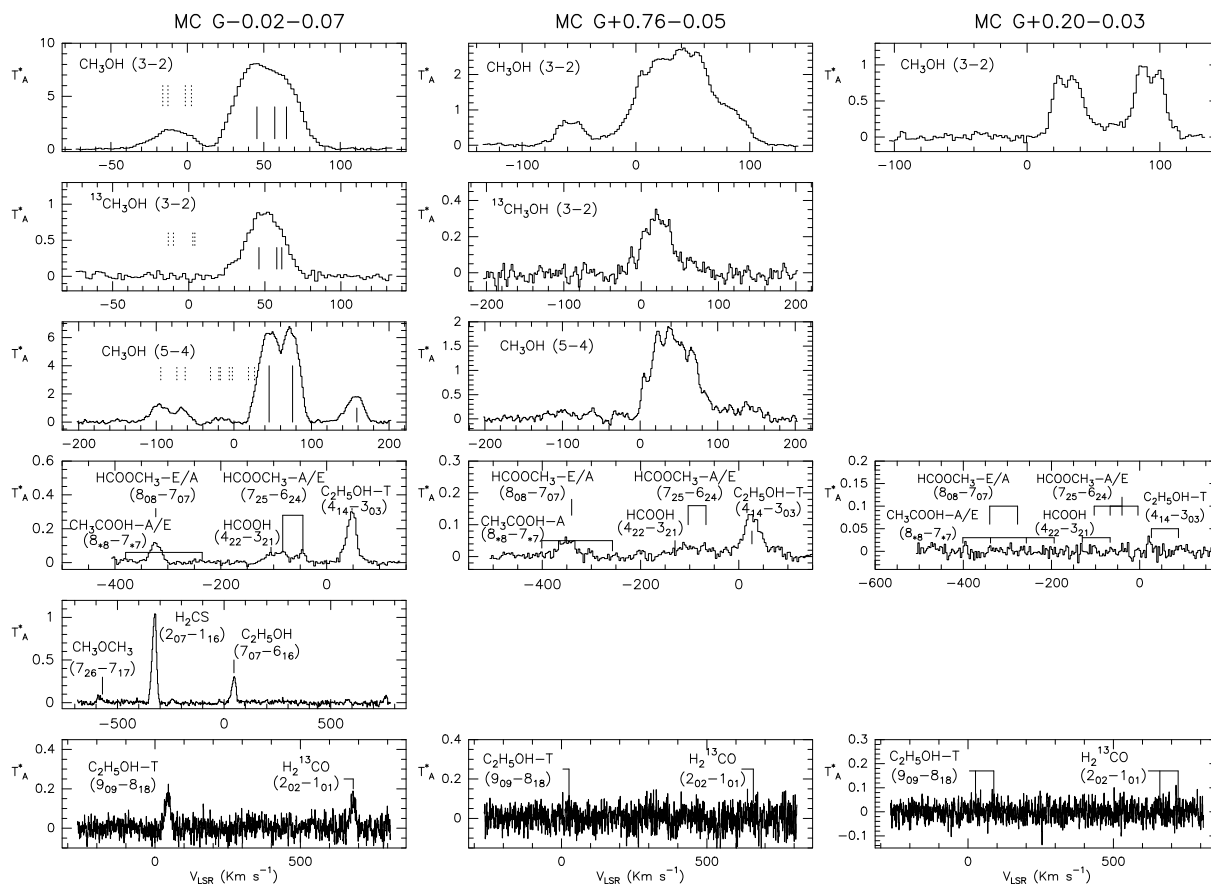
FIGURA 3.2: Perfiles típicos de las líneas observadas sobre tres de las fuentes del CG. En esta muestra se presentan los perfiles de las líneas de \text{CH}_3\text{OH} y de ^{13}\text{CH}_3\text{OH} que están compuestas de varias transiciones K_a de la molécula. Se muestran, para la fuente MC G-0.02-0.07, las posiciones para las transiciones más intensas en líneas sólidas verticales y las menos intensas con líneas de puntos verticales. En la fuente MC G+0.20-0.03 no se ha obtenido detección de ninguna molécula compleja excepto de \text{CH}_3\text{OH} , que presenta dos componentes en velocidad.
