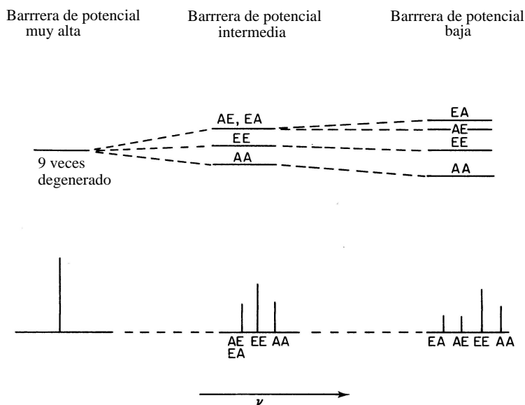
FIGURA A.6: División de un nivel rotacional por la rotación de dos rotores simétricos. Los niveles rotacionales se dividen en cuatro especies, que dependiendo de la barrera de potencial a la rotación se podrán ver separadas en el espectro o no. Figura adaptada de Lister et al. (1978).
