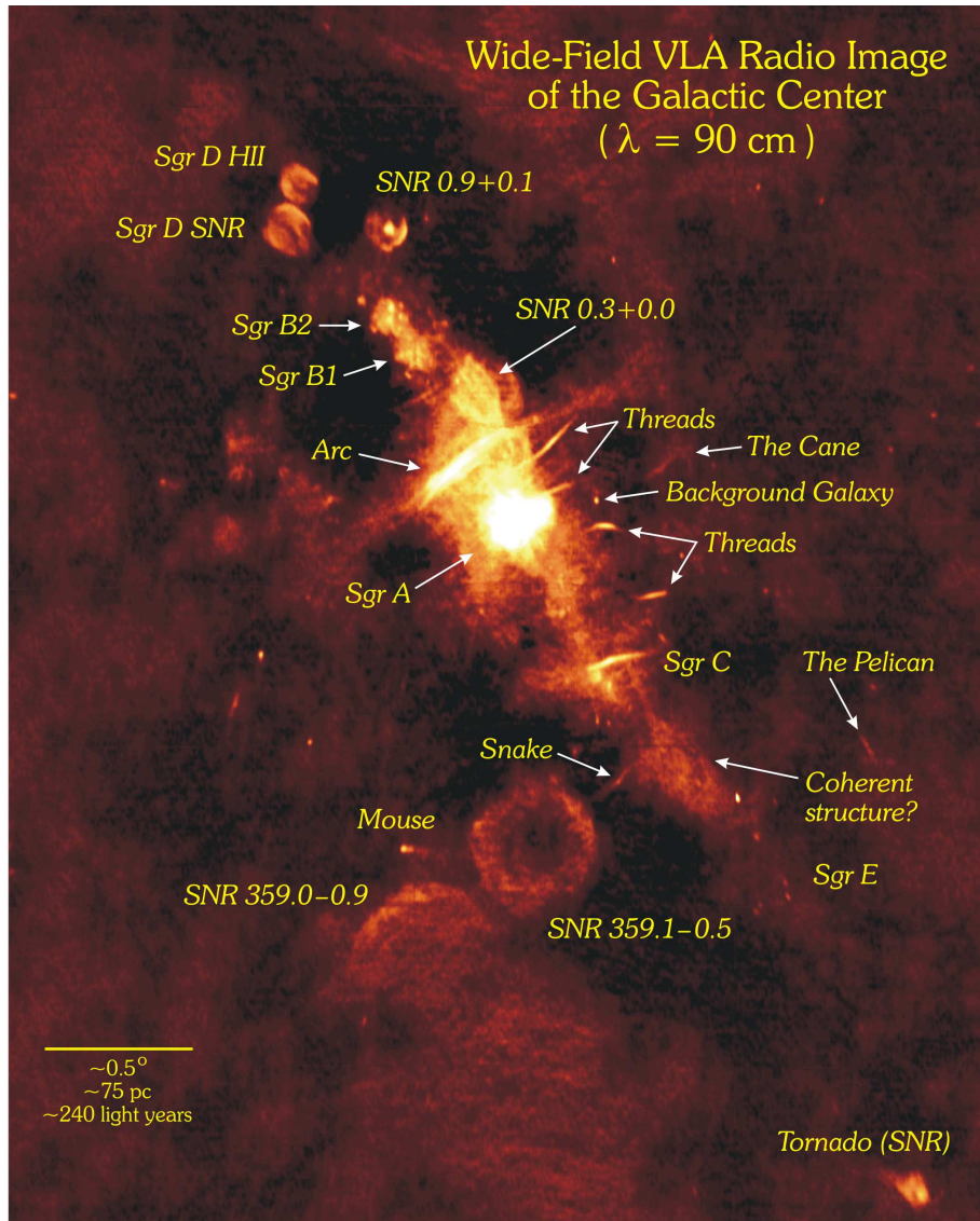
FIGURA 1.1: Mosaico de imágenes del continuo a 90 cm del CG obtenidas con el VLA. Figura de LaRosa et al. (2000).
