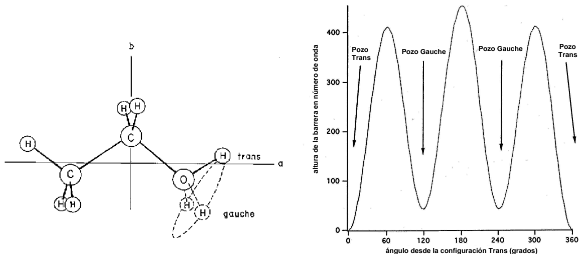
FIGURA A.11: Izq. Rotación del grupo OH del C_2H_5OH en la que se pueden ver las conformaciones Trans y Gauche. Drcha. Las barreras de potencial para el C_2H_5OH . Figuras de Zuckerman et al. (1975) y de Pearson et al. (1995).
