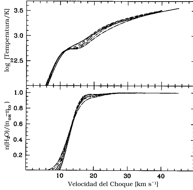
FIGURA 3.10: Temperatura que pueden alcanzar los choques tipo-C dependiendo de su velocidad para diferentes densidades de H_2 entre 10^4 – 10^{6.5} \text{ cm}^{-3} , la variación con la densidad no va a ser muy importante. Figura adaptada de Kaufman & Neufeld (1996).
