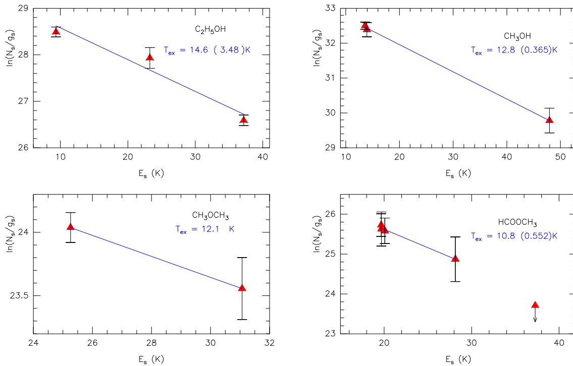
FIGURA 3.4: Diagramas de las poblaciones de los niveles de diferentes moléculas para la fuente MC G-0.02-0.07. En estos diagramas la inversa de la pendiente nos da la temperatura de excitación rotacional que se obtiene en esta región para cada una de las moléculas. Las barras de error se obtienen asumiendo un error en la calibración del 10%, típico del 30m, y del error del ajuste gaussiano. ( ) indican el error del ajuste y el triángulo con flecha indica el límite superior que se deriva de una transición.
