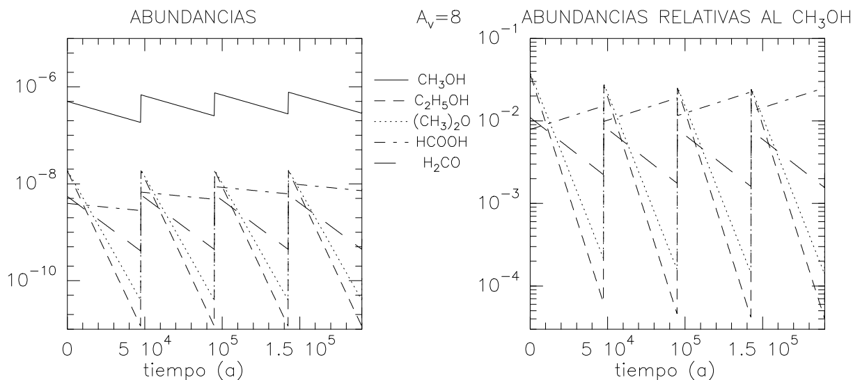
FIGURA 3.13: Abundancias y razones de abundancias de las MOCs en PDRs con A_v=8 con presencia de choques frecuentes cada 4.5 \times 10^4 años.
