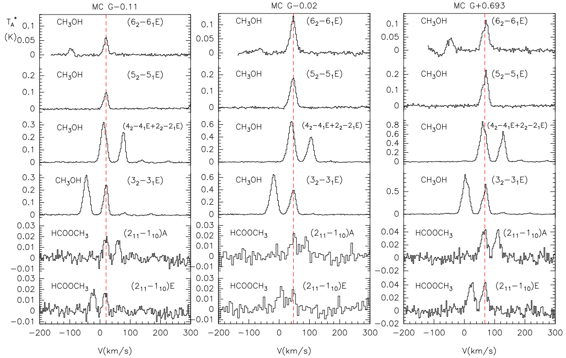
FIGURA 5.5: Perfiles espectrales de las transiciones de moléculas que ya se habían observado (ver Tab. 5.1).
