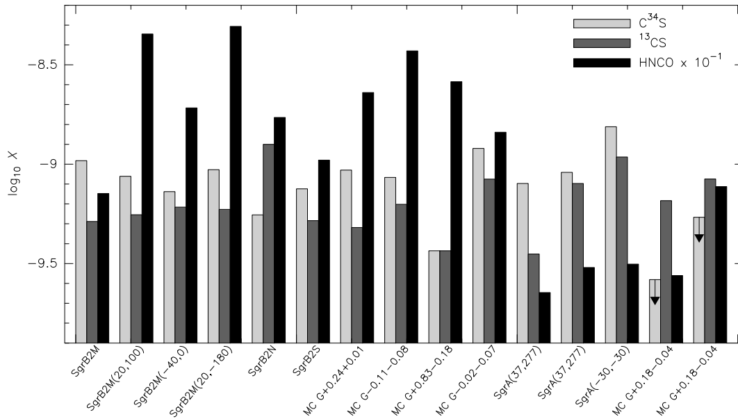
FIGURA 6.4: Abundancias relativas a H_2 asumiendo un factor de conversión de C^{18}O/H_2=4\times 10^{-7} . Las flechas representan límites superiores a las abundancias.
