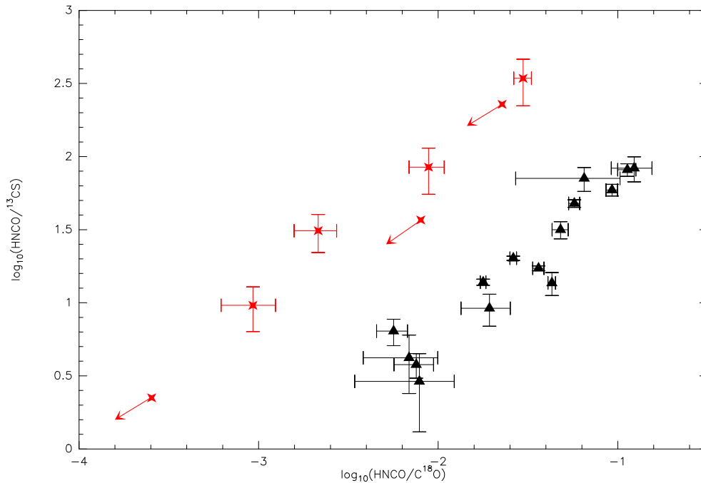
FIGURA 6.7: Razones de abundancia ^{13}\text{CS}/\text{HNCO} respecto a la razón \text{C}^{18}\text{O}/\text{HNCO} en escala logarítmica para la muestra de fuentes observadas en el centro Galáctico y para las galaxias que se presentan en la Tab. 6.5. Los triángulos representan las nubes del CG y las estrellas las galaxias, en dos de ellas sólo se han derivado límites en la densidad de columna de \text{HNCO} y se muestra con la flecha la dirección del límite.
