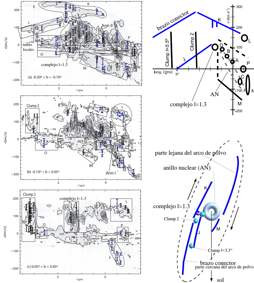
FIGURA 1.8: Izq: Diagramas de la velocidad respecto a la longitud galáctica para diferentes rangos de latitud galáctica de la emisión de CO(1-0). En estas figuras se marcan los principales complejos moleculares que a continuación podremos ver distribuidos en los esquemas de la derecha. Drcha. Arriba: Esquema que ilustra todas los complejos moleculares. Las letras de la A a la D representan los complejos moleculares Sgr A–Sgr D. Drcha. Abajo: Esquema de la distribución de las nubes moleculares que se comentaban anteriormente con respecto a la línea de mira. Figuras adaptadas de Rodríguez-Fernández et al. (2006).
