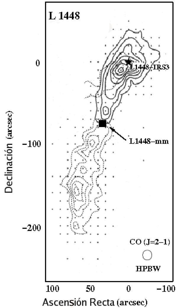
FIGURA 4.2: Distribución del CO ( J=2 \rightarrow 1 ) en la nube molecular L1448. En esta figura se puede observar el flujo bipolar L1448-mm. Figura adaptada de Bachiller et al. (1990).
