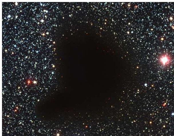
FIGURA 2.1: Nube oscura Barnard 68 observada en el óptico. Figura de Herbst (2001).
