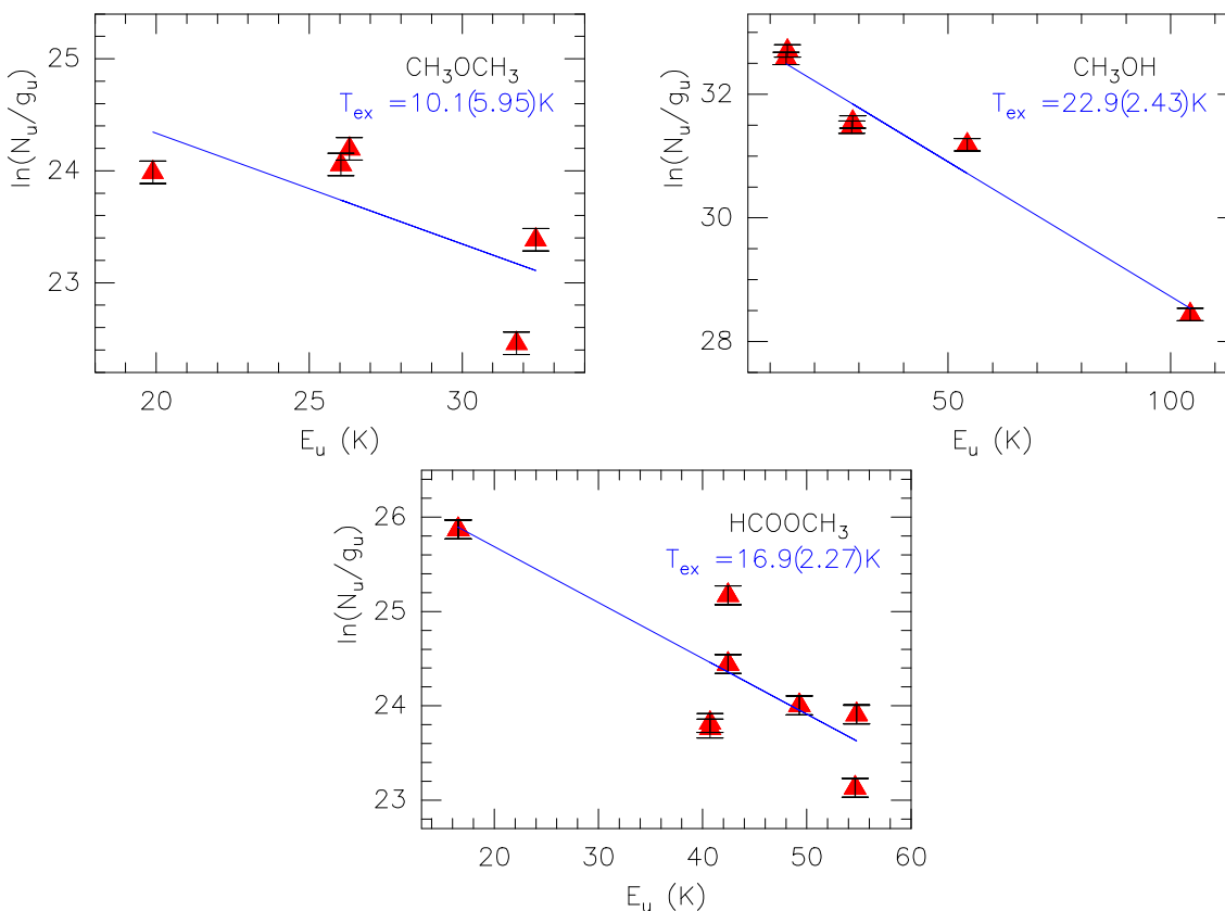
FIGURA 3.5: Diagramas de poblaciones de niveles para algunas moléculas complejas en MC G-0.02-0.07 derivados de datos de Martín (2006a). Ver Fig. 3.4.
