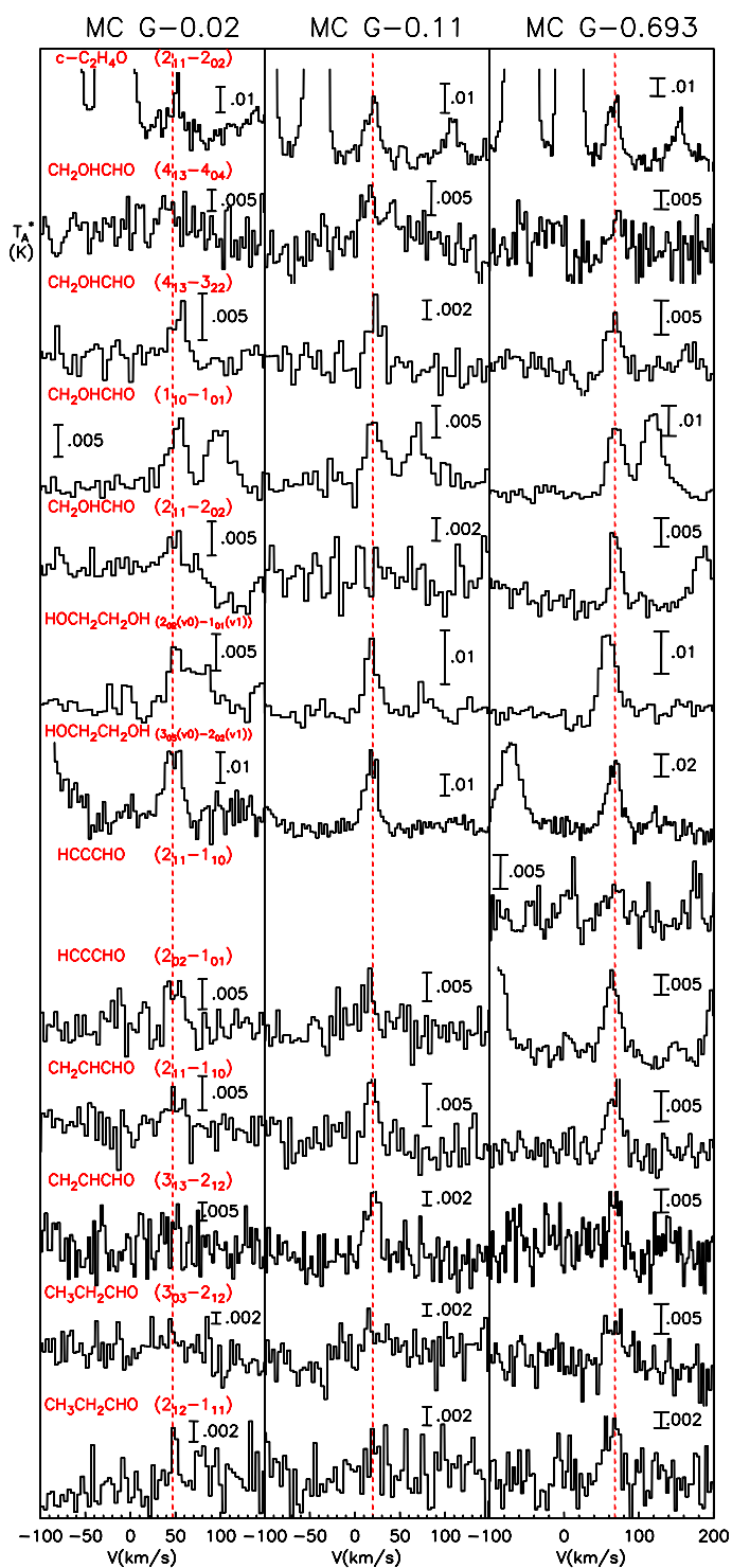
FIGURA 5.4: Espectros de las nuevas transiciones moleculares que han sido observadas (ver Tab. 5.1) en las tres fuentes del CG. MC G+0.693 es la fuente con más detecciones. Las líneas verticales marcan las velocidades de las nubes, a 20 \text{ km s}^{-1} para MC G-0.11, a 49 \text{ km s}^{-1} para MC G-0.02 y a 68 \text{ km s}^{-1} para MC G+0.693.
