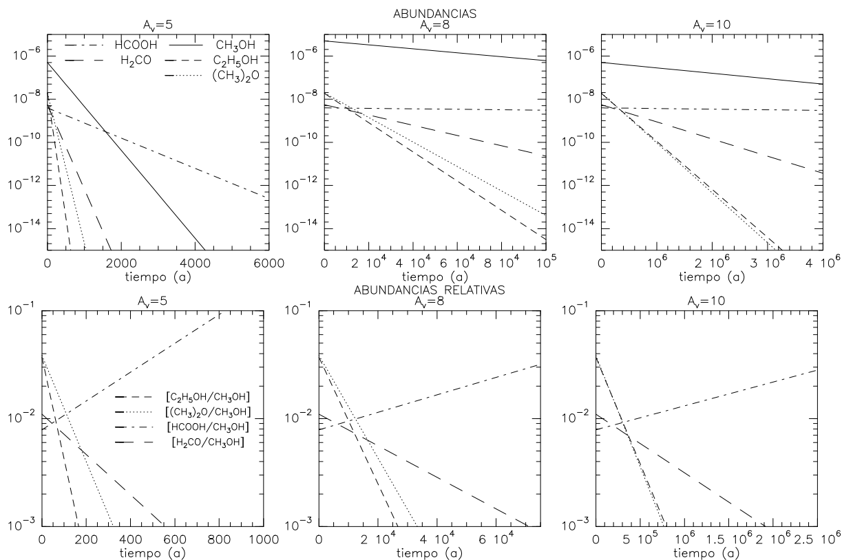
FIGURA 3.12: Abundancias y razones de abundancias de las MOCs con respecto a \text{CH}_3\text{OH} en regiones de foto-disociación.
