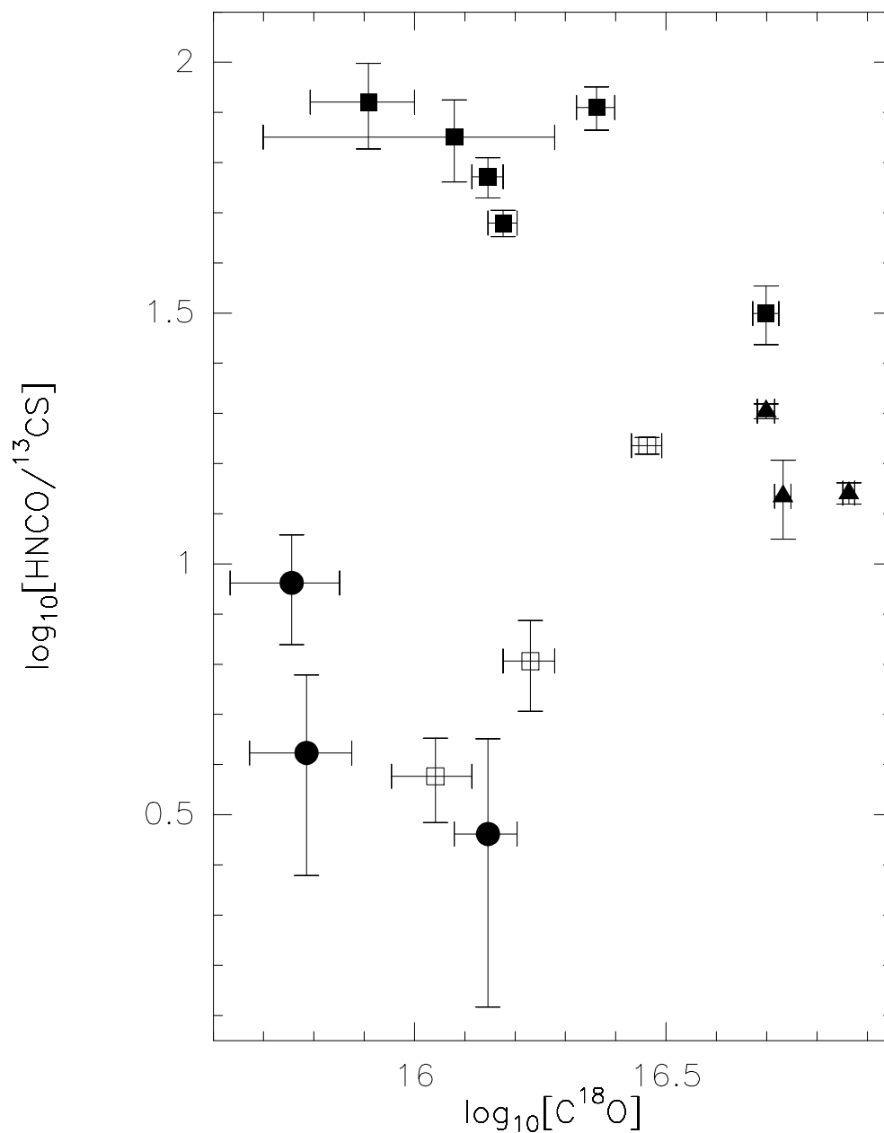
FIGURA 6.5: Razón de abundancias ^{13}\text{CS}/\text{HNCO} respecto a la densidad de columna de \text{C}^{18}\text{O} en escala logarítmica para la muestra de fuentes observadas en el centro Galáctico. Los círculos rellenos representan las nubes donde domina la radiación UV, los cuadrados vacíos las regiones afectadas por choques de tipo-J, los cuadrados rellenos las nubes moleculares típicas del centro Galáctico, los triángulos los núcleos calientes.
