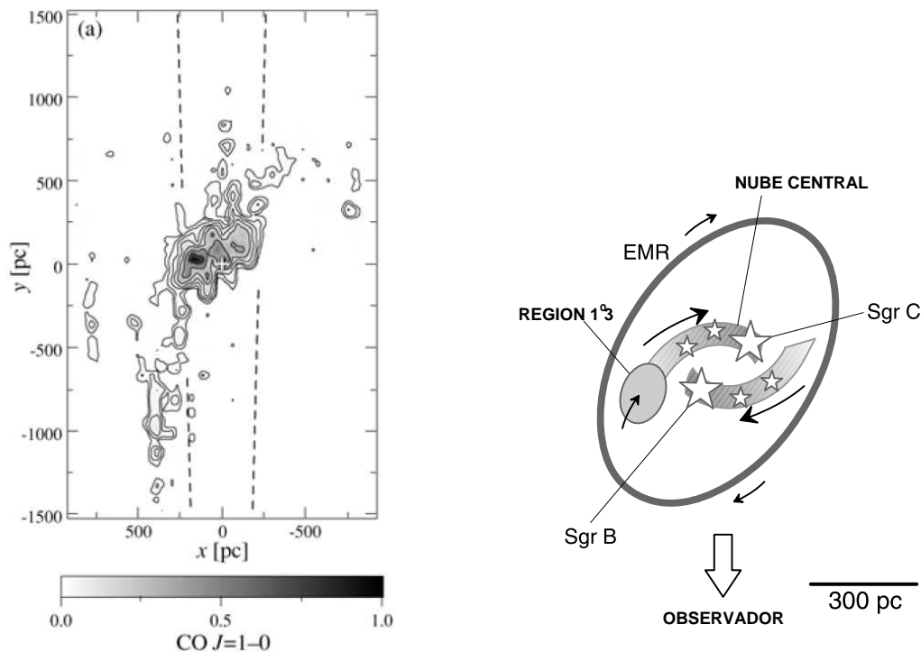
FIGURA 1.7: Izq: Disposición de las nubes del CG a lo largo de la línea de mira obtenidas a partir de observaciones de CO y de OH. Dcha: Esquema de la distribución de los complejos de nubes en la zona interna del CG. Figuras de Sawada et al. (2004).
