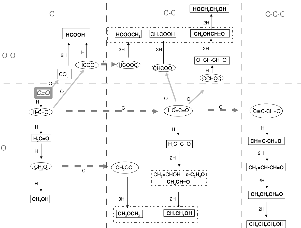
FIGURA 5.8: Posibles rutas de formación de MOCs en la superficie de los mantos de los granos. La complejidad química va aumentando de izquierda a derecha al añadir C, desde el centro hacia arriba y hacia abajo añadiendo H y en diagonal añadiendo O. Los radicales se presentan dentro de elipses y las moléculas neutras dentro de cajas. Las moléculas en negrita son las que se han observado en la ZMC en este trabajo. Las otras moléculas no han sido detectadas todavía o sus parámetros espectroscópicos no se han estudiado. Por último se muestran en las familias de isómeros en cajas discontinuas. Esta figura está adaptada de Charnley & Rodgers (2005) y Tielens & Hagen (1982).
