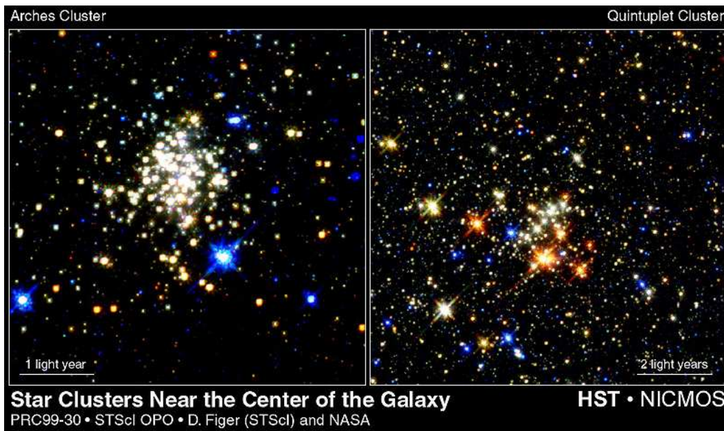
FIGURA 1.4: Cúmulos de Los Arcos y del Quintuplete.
