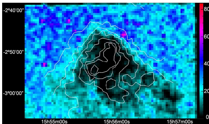
FIGURA 4.1: Imagen que muestra el conteo de estrellas en la región de L183 en la banda I. Y superpuesto los contornos de Isophot a 200\mu\text{m} . En las zonas más internas de la nube molecular no se observa ninguna estrella. Referencia de Pagani et al. (2005).
