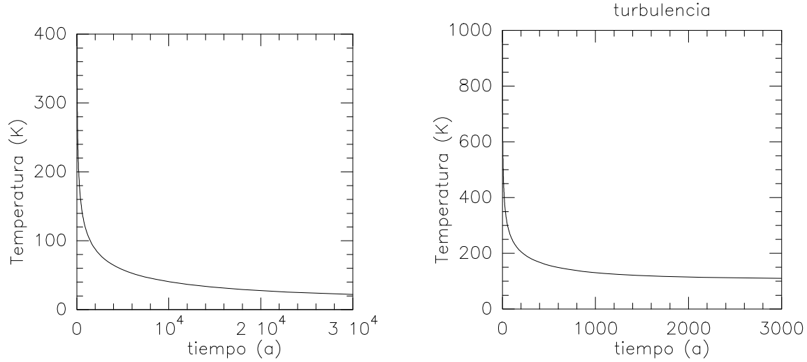
FIGURA 3.11: Enfriamiento tras un choque tipo-C a 15 \text{ km s}^{-1} en un medio con densidades de 10^5 \text{ cm}^{-3} . En la figura de la izquierda no se introduce el calentamiento debido a la turbulencia, mientras que en la figura de la derecha sí.
