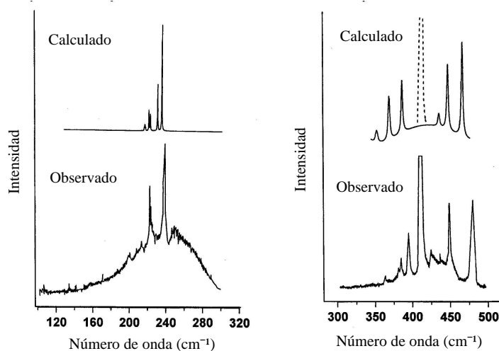
FIGURA A.14: Espectro obtenido a partir de cálculos ab initio sin tener en cuenta las fuerzas estéricas (líneas continuas en la parte superior de los paneles), comparado con el observado (parte inferior de los paneles). En el panel de la izquierda se observa que la posición en número de ondas de las líneas calculadas no concuerda con las observadas. En el panel de la derecha se puede ver como se pierden líneas espectrales. La línea punteada aparece al introducir las fuerzas estéricas. Figura de Senent et al. (1995).
