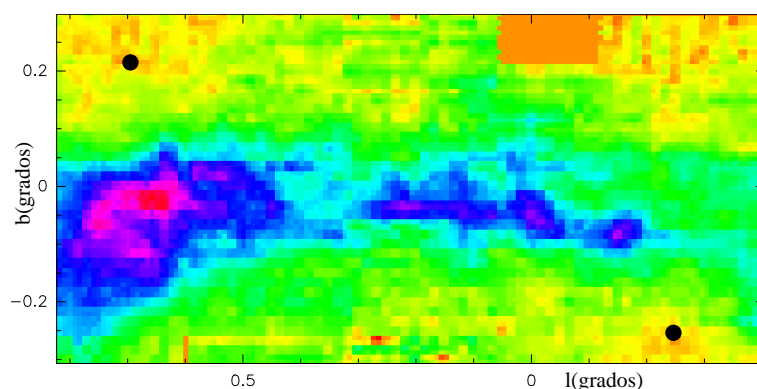
FIGURA 5.3: Mapa de la ZMC de la emisión de CS de Bally et al. (1987). Cuanto más oscuro más intensa la emisión. Los puntos negros marcan las posiciones de referencia utilizadas en la observación, la emisión en estas posiciones es mínima.
