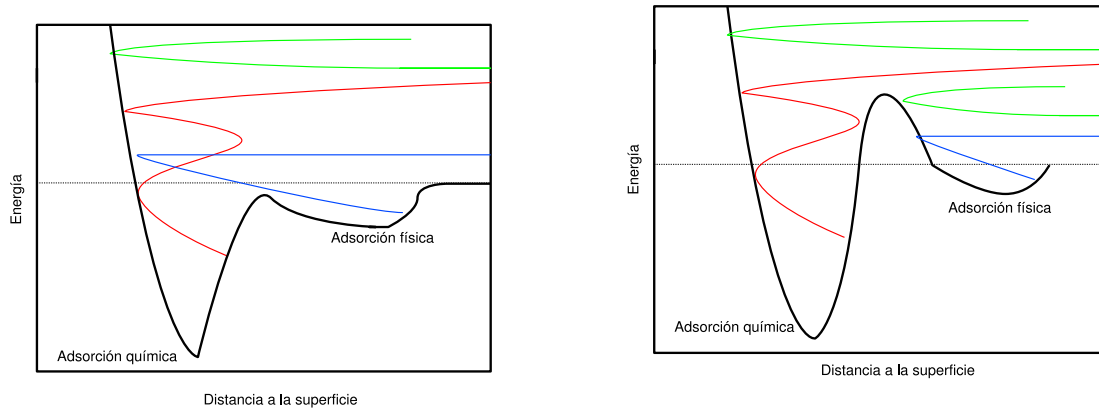
FIGURA 2.3: Pegado o no pegado según la energía relativa y el potencial.
