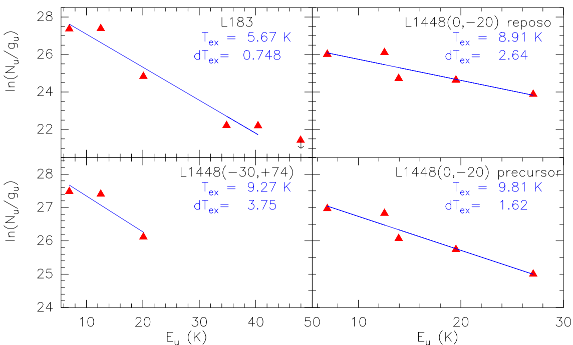
FIGURA 4.4: Diagramas de poblaciones de los niveles de \text{CH}_3\text{OH} en L183, L1448 ( 0'' , -20'' ) (para las dos componentes, gas en reposo y precursor) y en L1448 ( -30'' , +74'' ).
